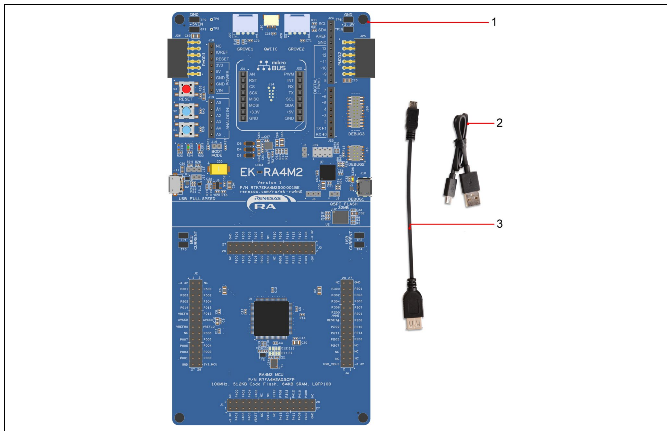
図 1 EK-RA4M2 評価キット構成
