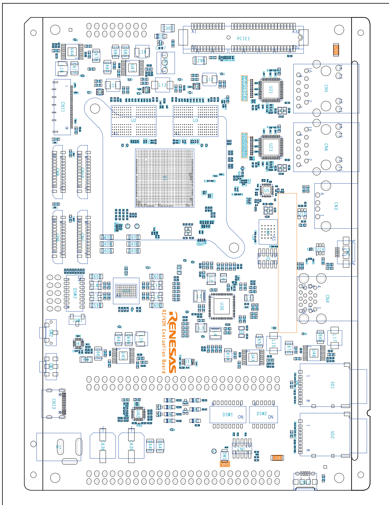
付録 A.1 部品配置図 (Top)
