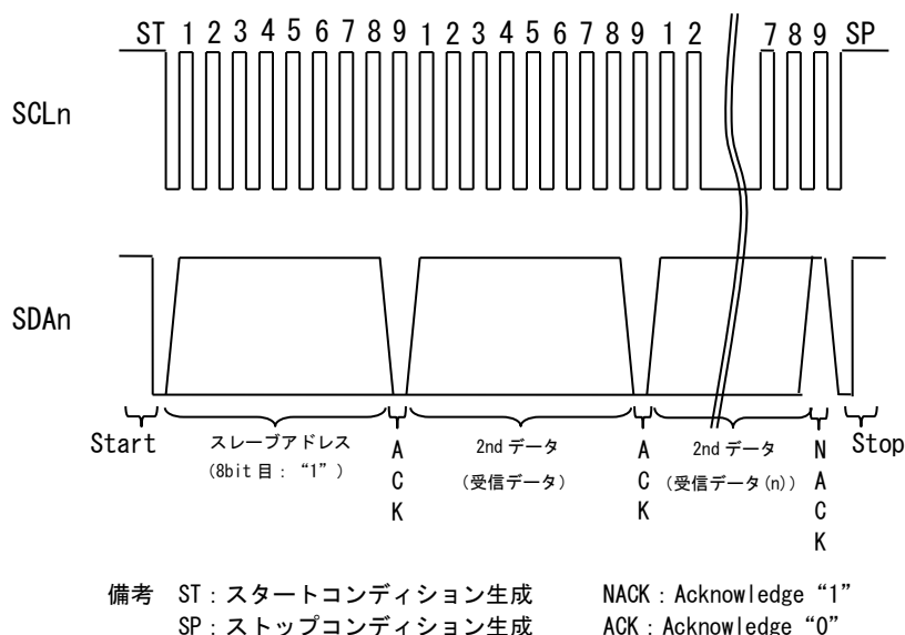
図 6-6 マスタ受信 信号図
