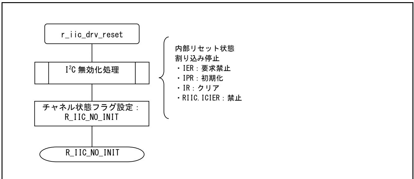
図 6-31 I 2 C ドライバリセット関数概略フロー
