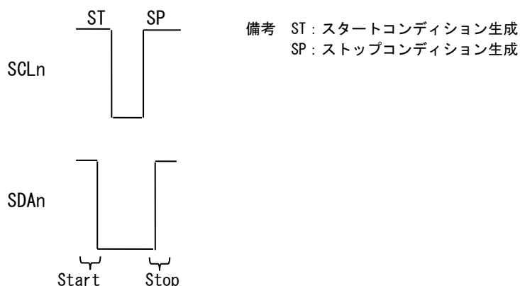
図 6-5 マスタ送信（パターン 4 動作）信号図
