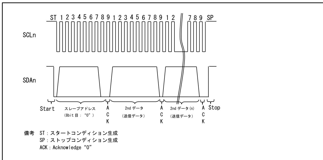
図 6-3 マスタ送信 (パターン 2) 信号図
