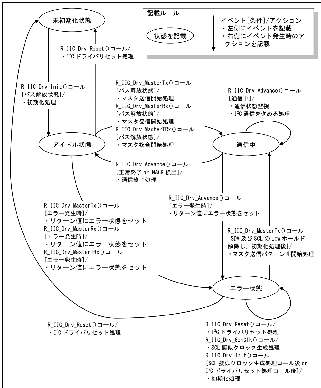
図 6-15 状態遷移図
